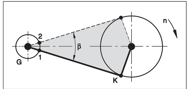
Rys. 5: Kąt obrotu \beta w mechanizmie korbowym
